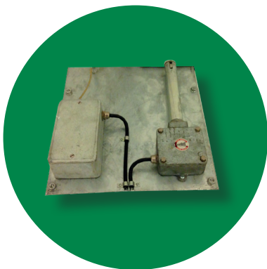
Schmelzlot- und Druckwellensystem
