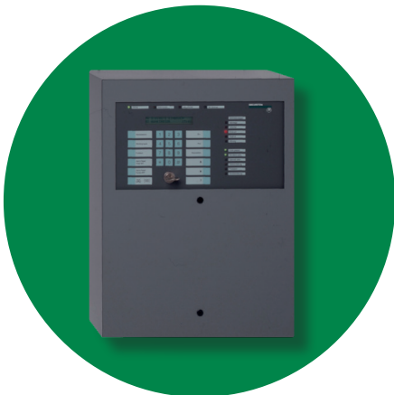
Einbruchmeldesystem Master Slave (SMS)
